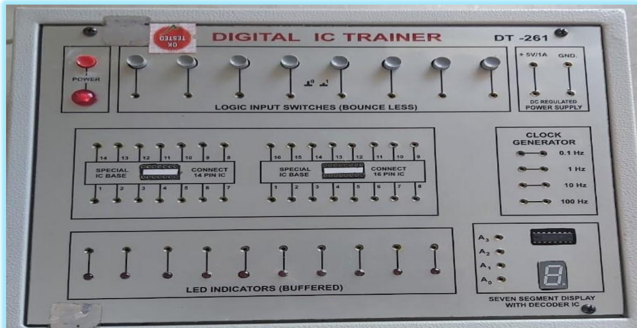
DIGITAL IC TRAINER
